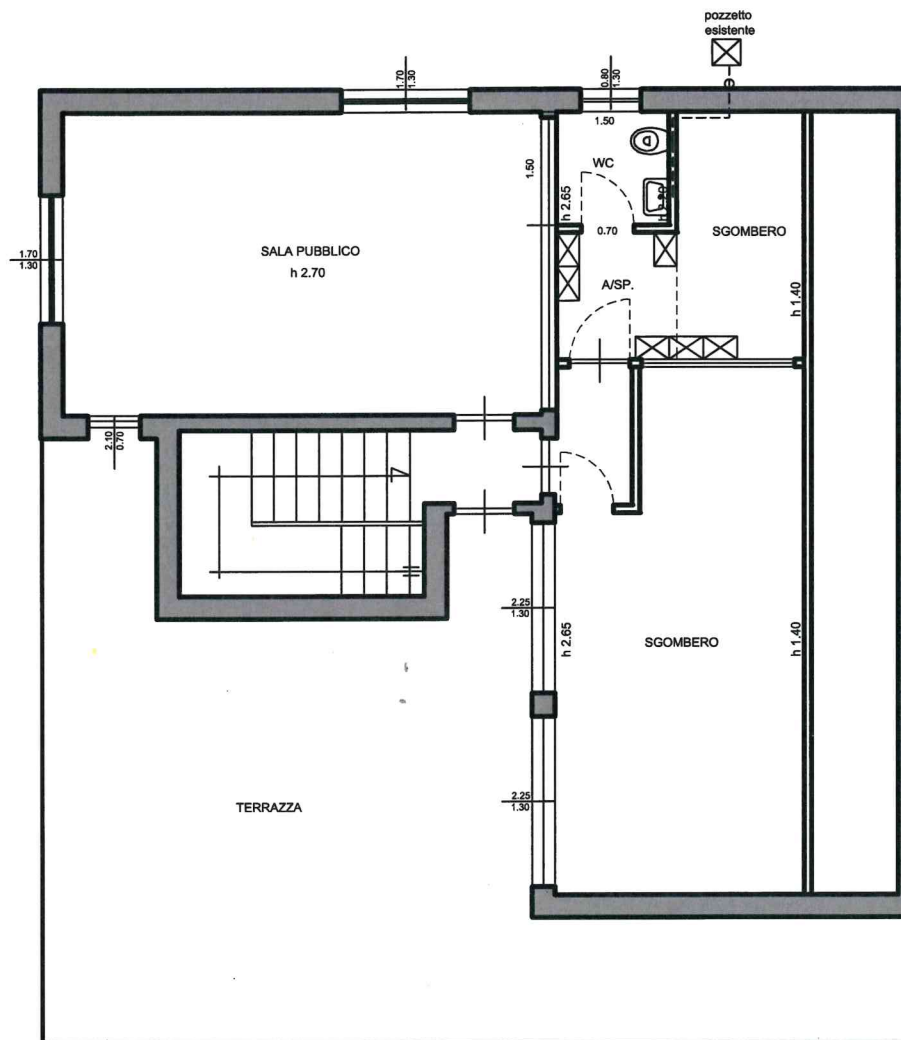
PIANO PRIMO
