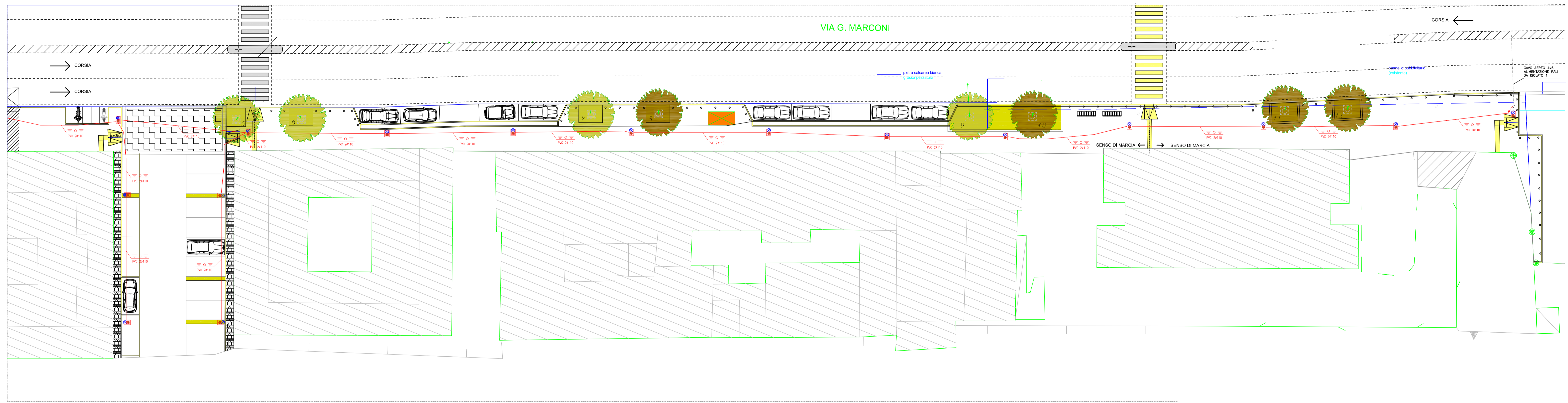
PLANIMETRIA LATO MARE - DIREZIONE STAZIONE SCALA 1:200
