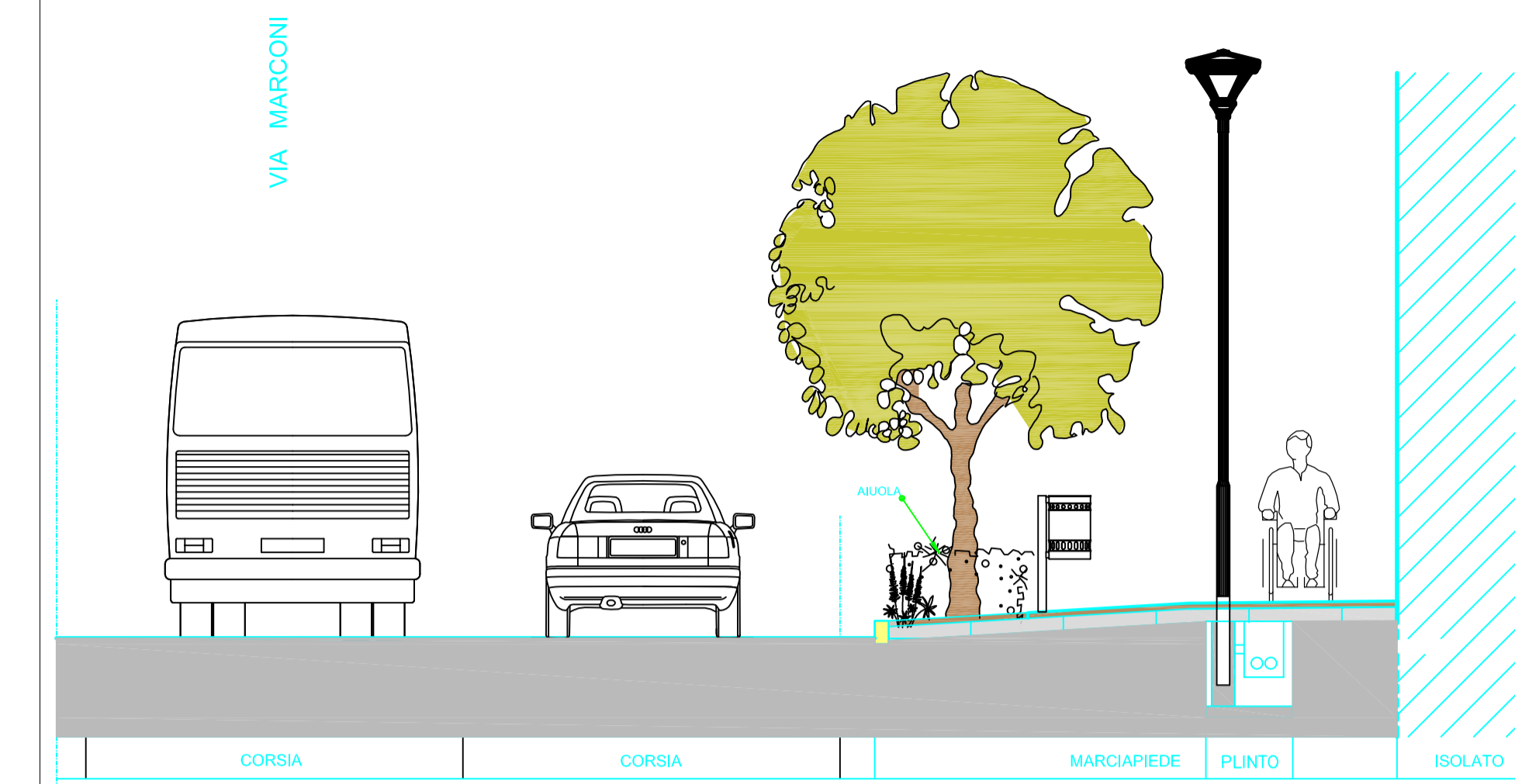
SCALA 1:50
