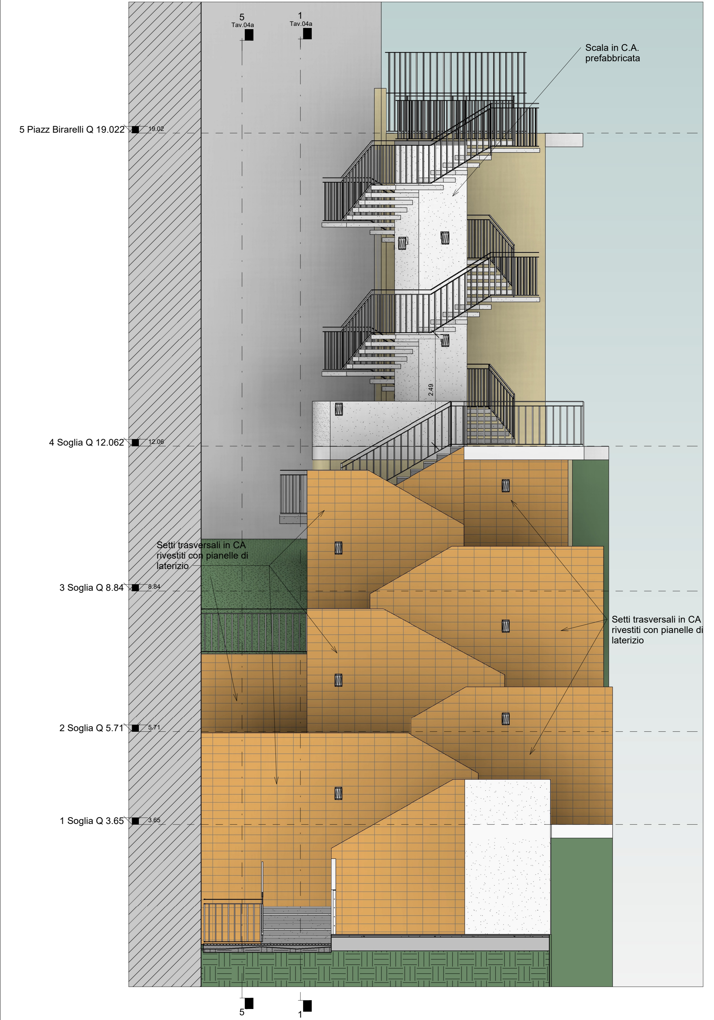
Prospetto Frontale
