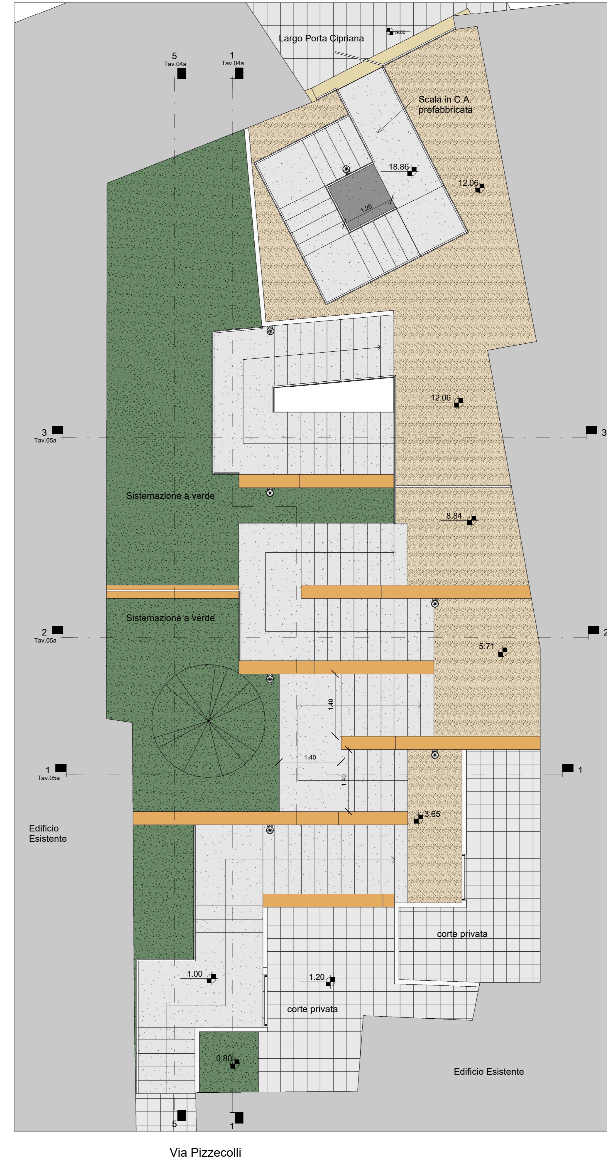
Pianta Generale
