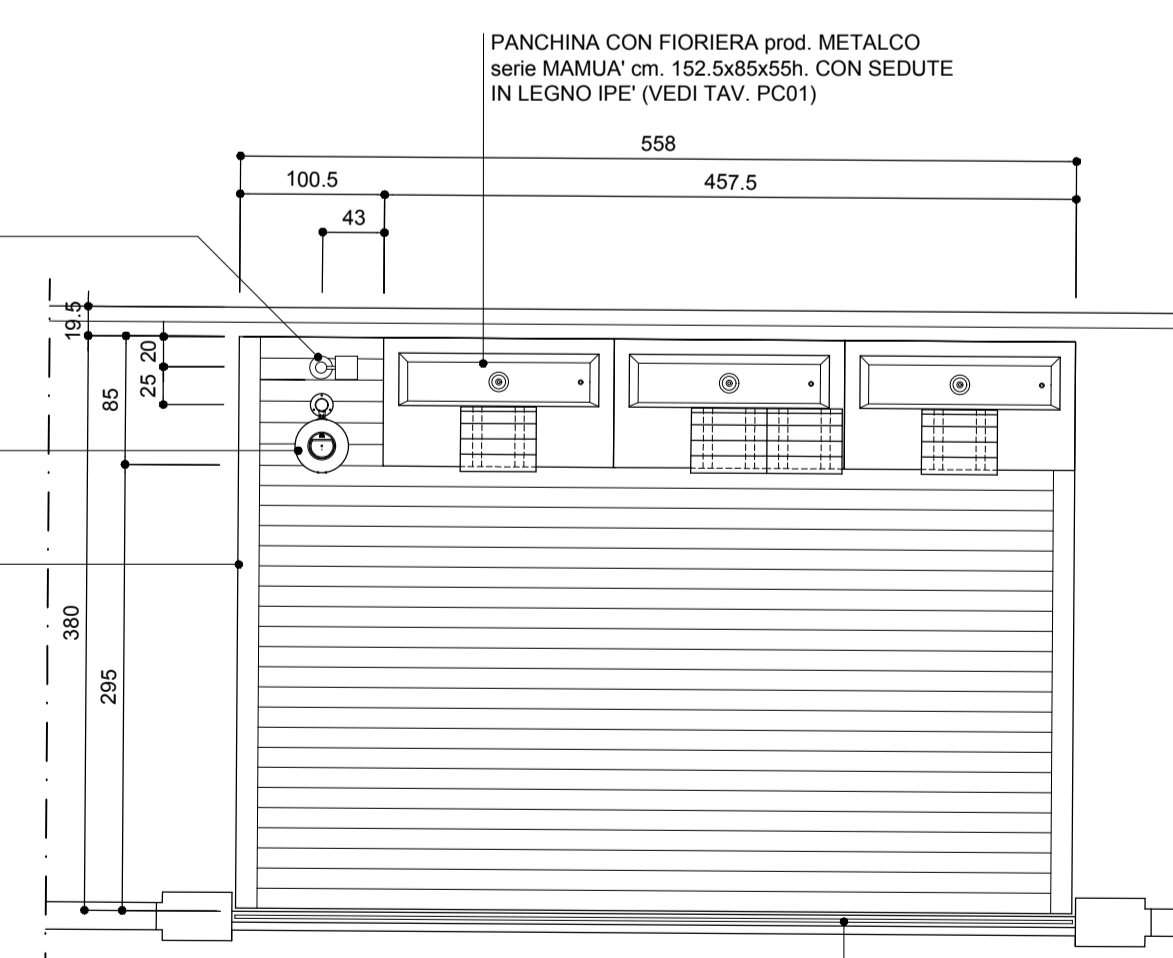
PEDANA IN LEGNO ⑤ PIANTA - RAPP. 1: 50
