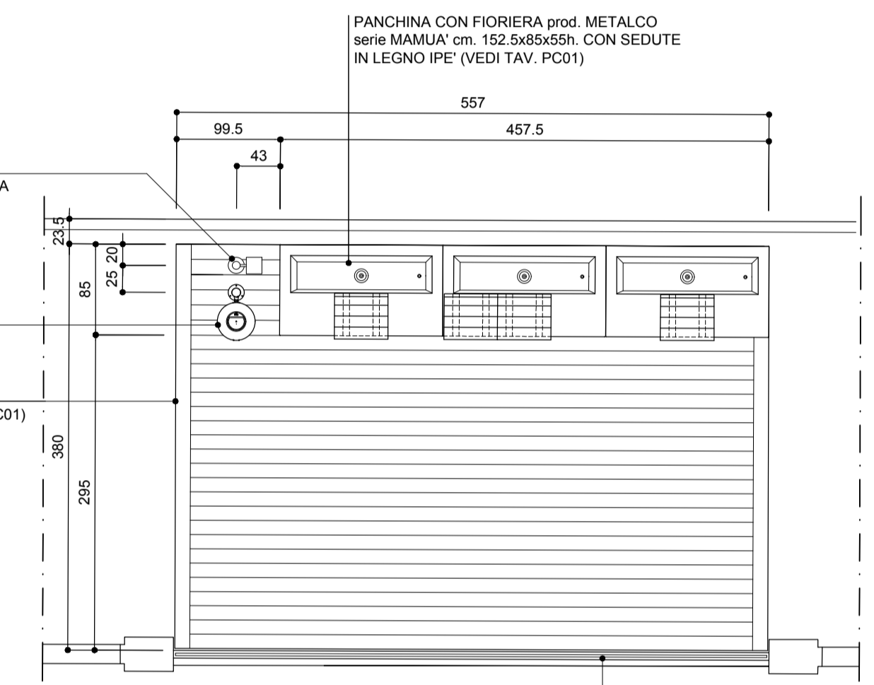
PEDANA IN LEGNO ③ PIANTA - RAPP. 1: 50
