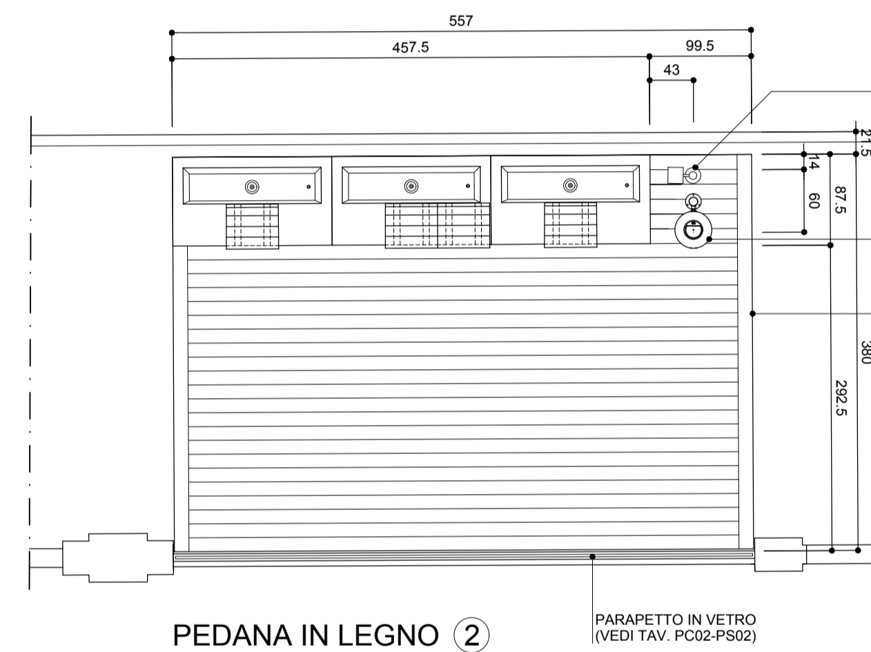
PEDANA IN LEGNO ② PIANTA - RAPP. 1: 50
