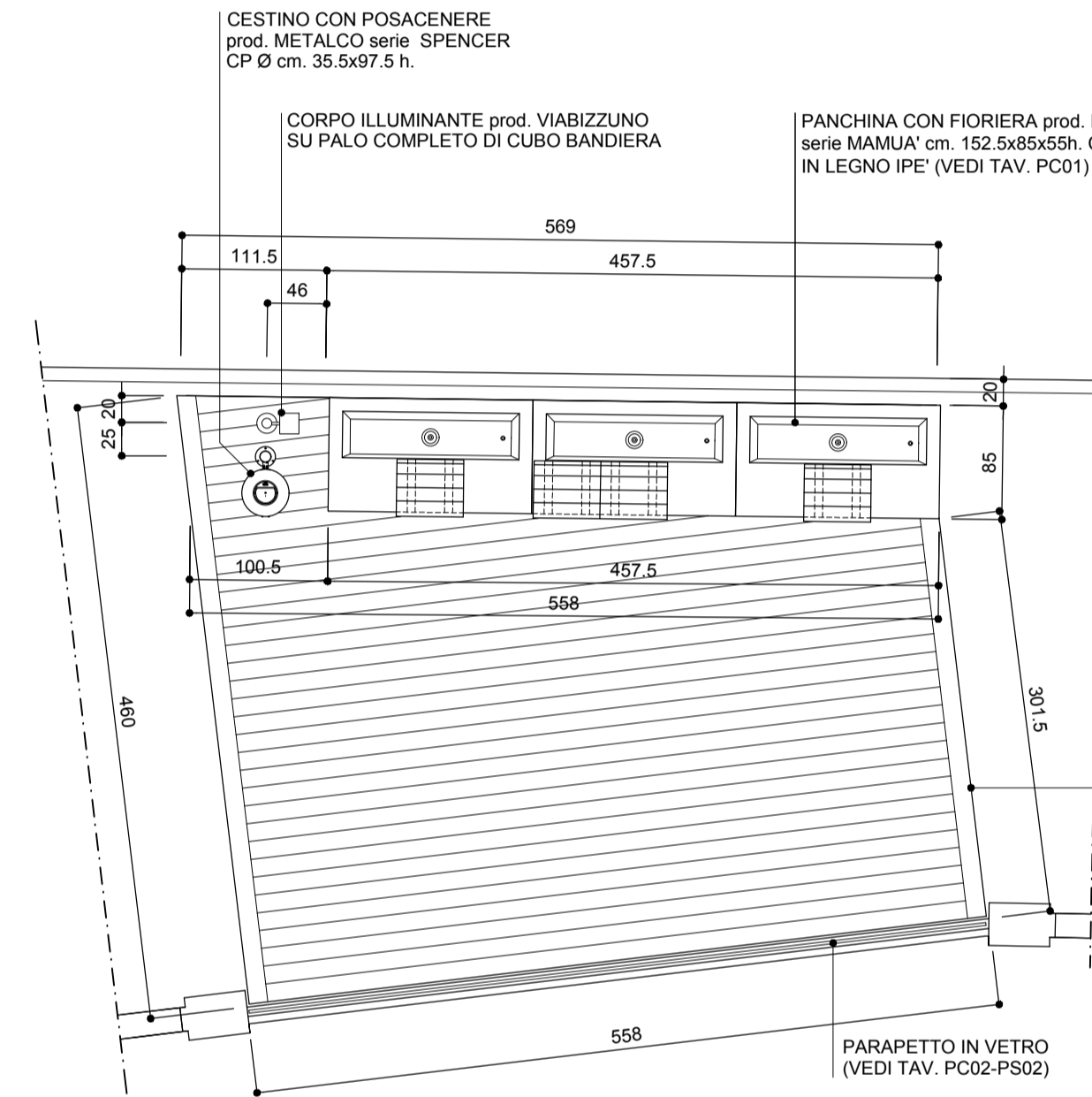
PEDANA IN LEGNO ① PIANTA - RAPP. 1: 50
