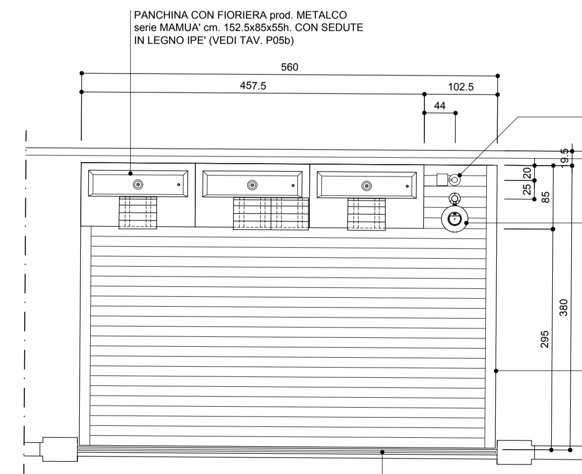
PEDANA IN LEGNO ④ PIANTA - RAPP. 1: 50
