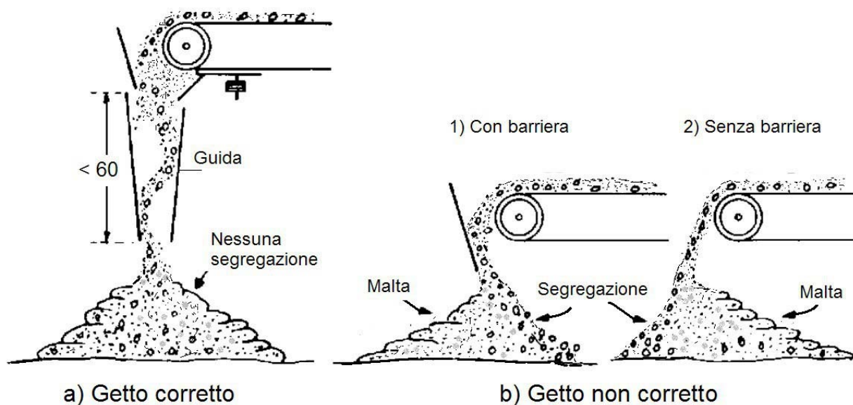
Figura - Esempi di getto di calcestruzzo con nastro trasportatore: a) getto corretto e b) getto non corretto. Nel caso b) si ha la separazione degli aggregati dalla malta cementizia. La barriera comporta soltanto il cambiamento di direzione della segregazione.
