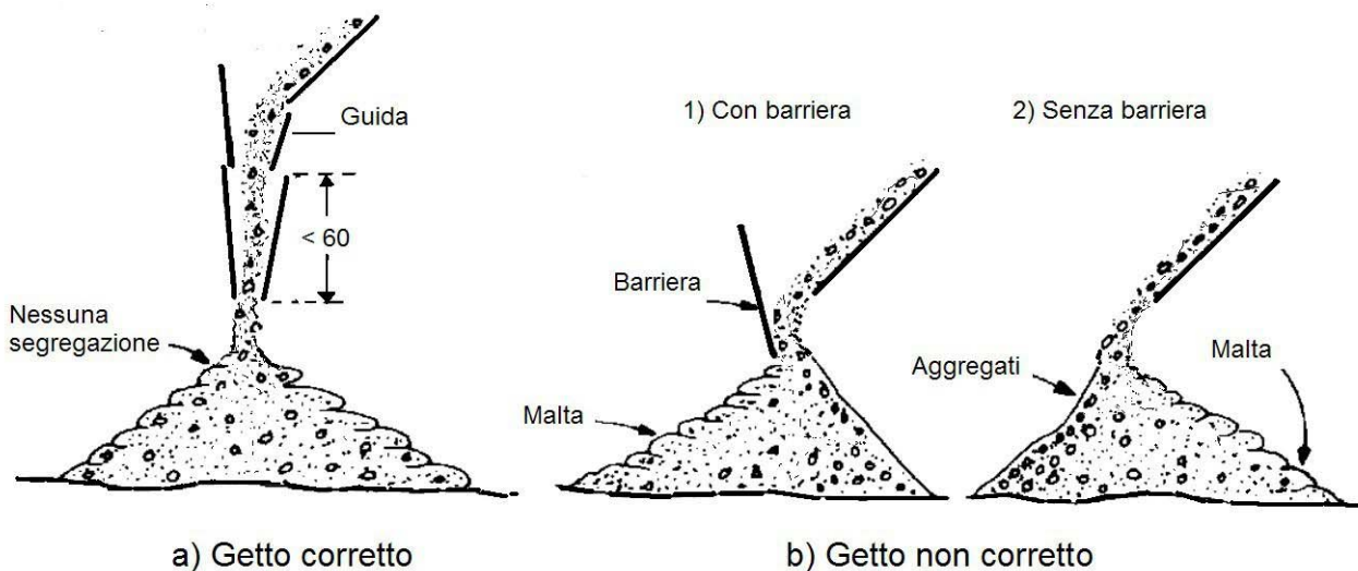
Figura - Esempi di getto di calcestruzzo da piano inclinato: a) getto corretto e b) getto non corretto. Nel caso b) si ha la separazione degli aggregati dalla malta cementizia. La barriera comporta soltanto il cambiamento di direzione della segregazione.
