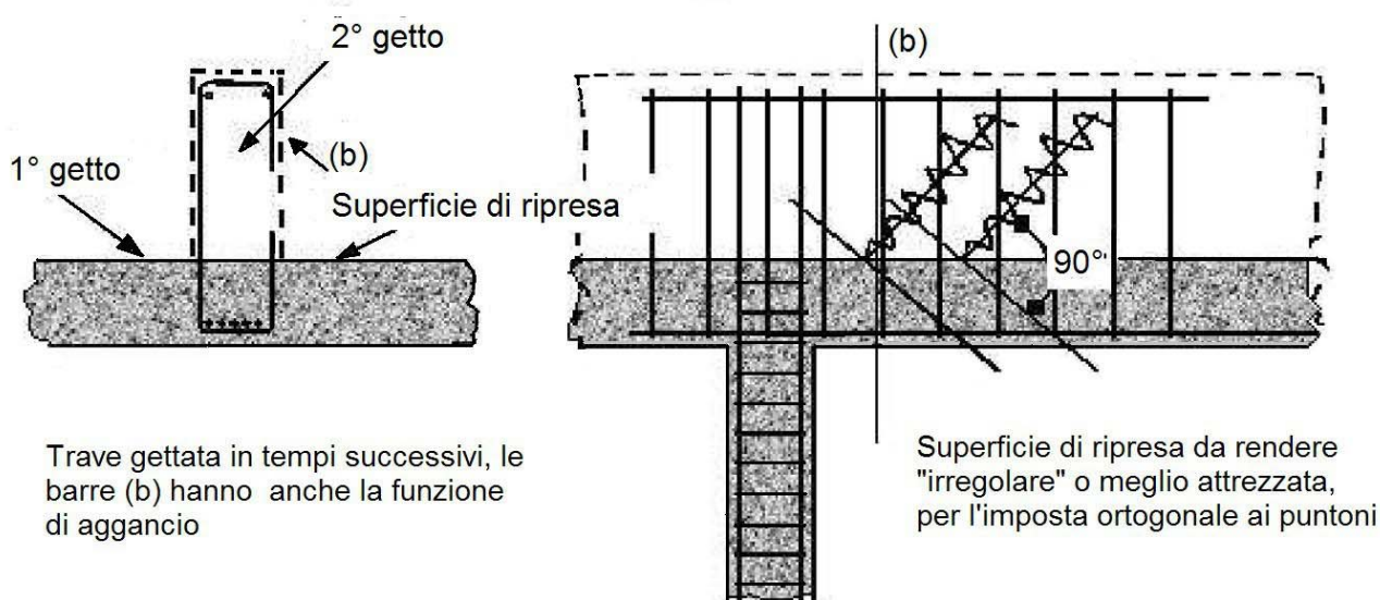
Figura - Modalità di ripresa del getto su travi di spessore elevato
