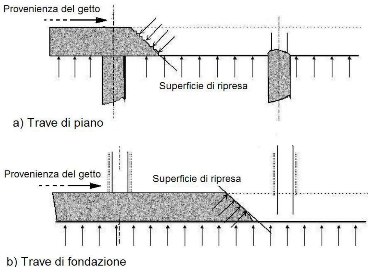
Figura - Modalità di ripresa del getto in travi di piano e di fondazione
