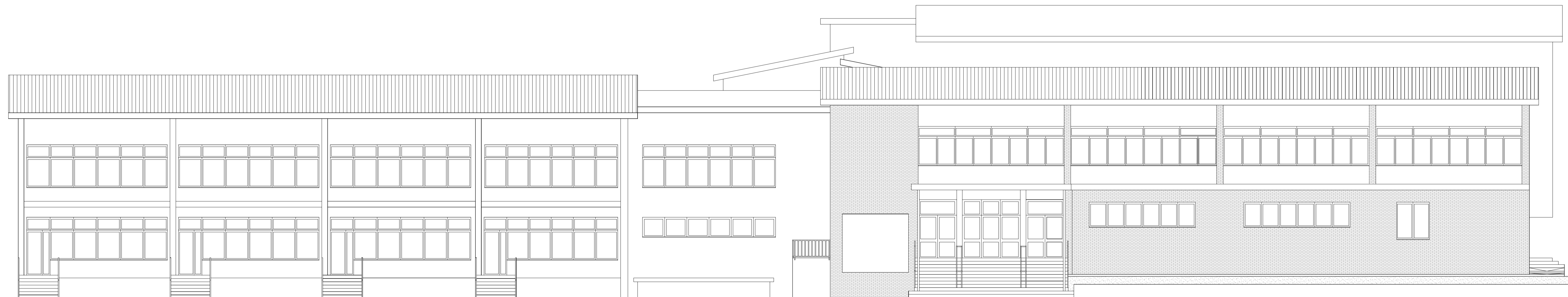
PROSPETTO SUD OVEST - CORPO B
