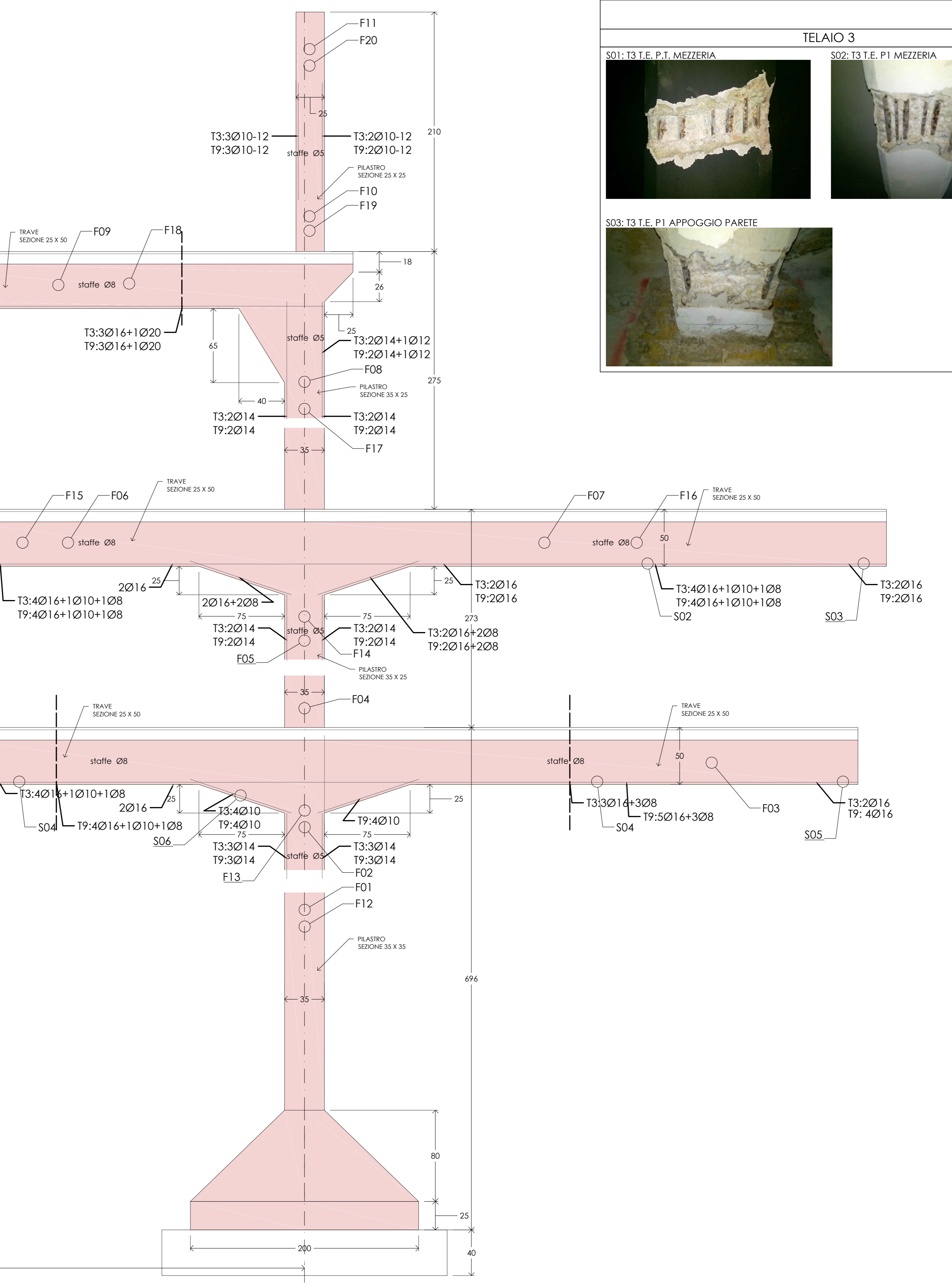
- INDAGINI PACOMETRICHE SUI TELAI 3 E 9 DELLA STRUTTURA "NERVI" - (scala 1:20)
