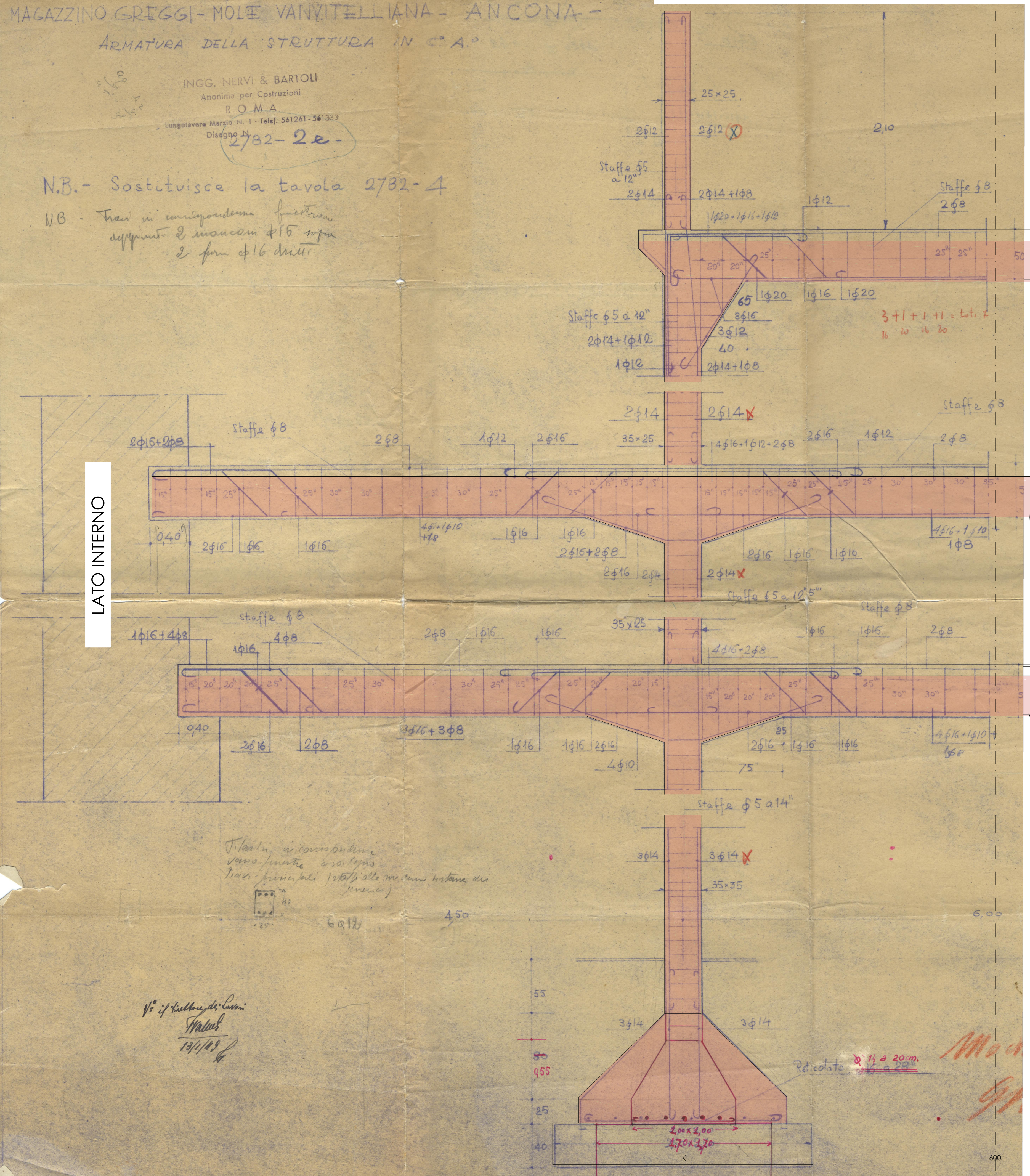
- INDAGINI PACOMETRICHE SUI TELAI 3 E 9 DELLA STRUTTURA "NERVI" - (scala 1:20)
