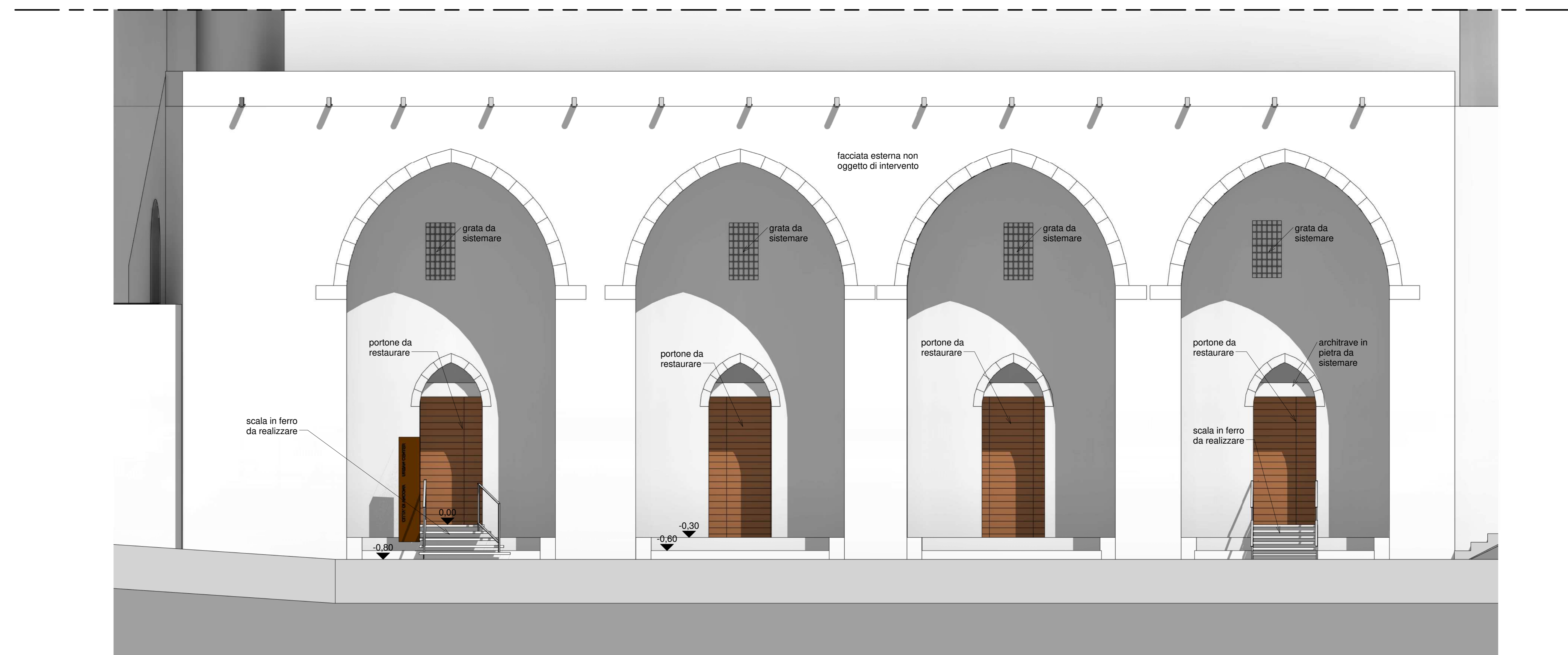
Prospetto Frontale
