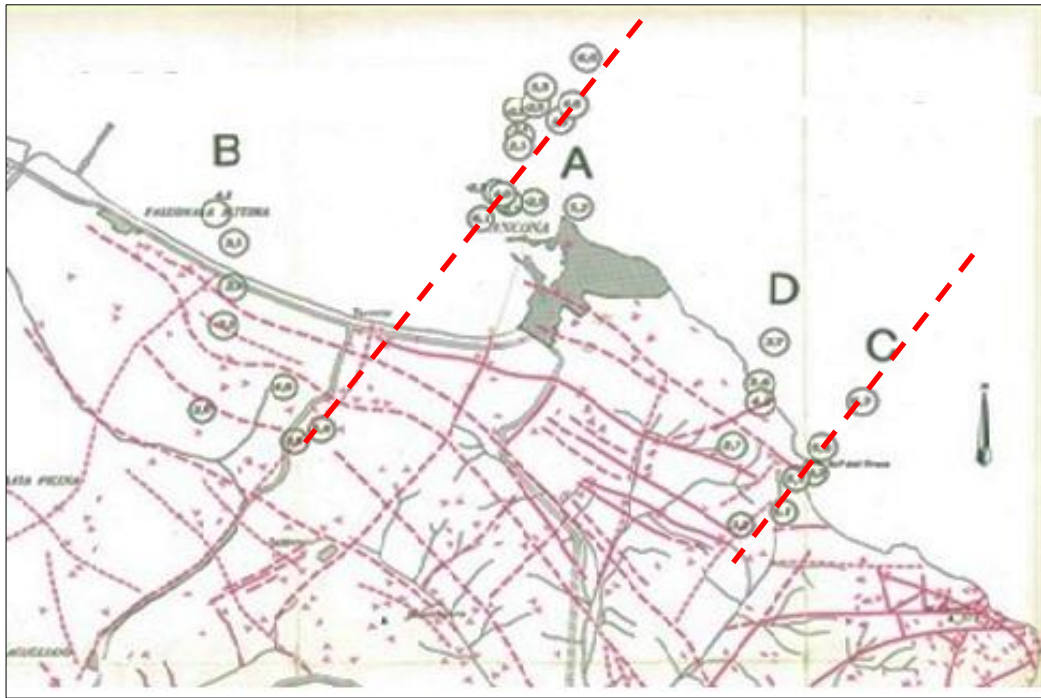
Fig. 2.5 Mappa degli epicentri con relative profondità – eventi dal 1972 al 1976 (Crescenti 1978).
