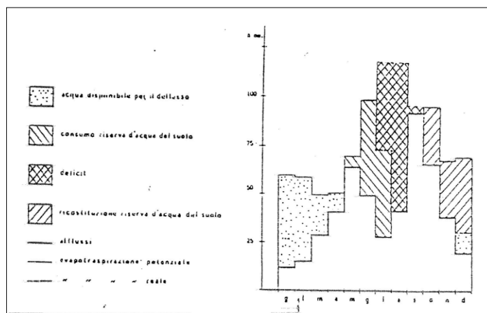
Fig. 3.5 - Bilancio idrologico secondo Thornthwaite
