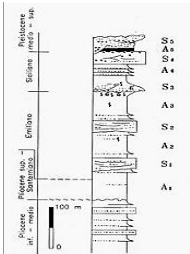
Fig. 3.2: Schema riassuntivo dei cicli del pleistocene
