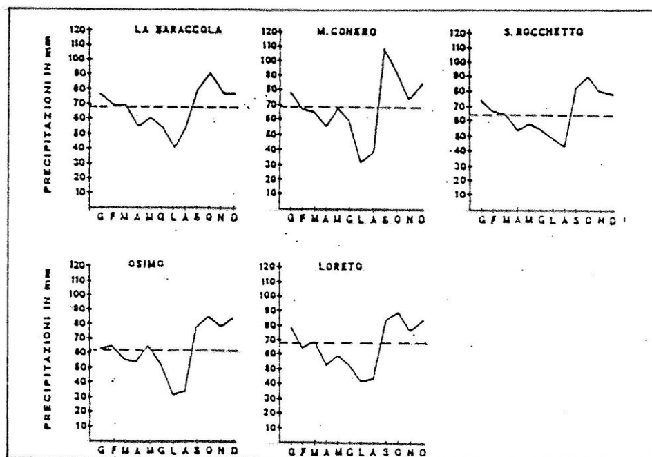
Fig. 3.4 - Diagrammi Pluviometrici
